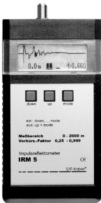
Impulsreflektometer
